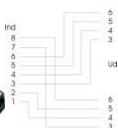
2x4 trådsadapter
